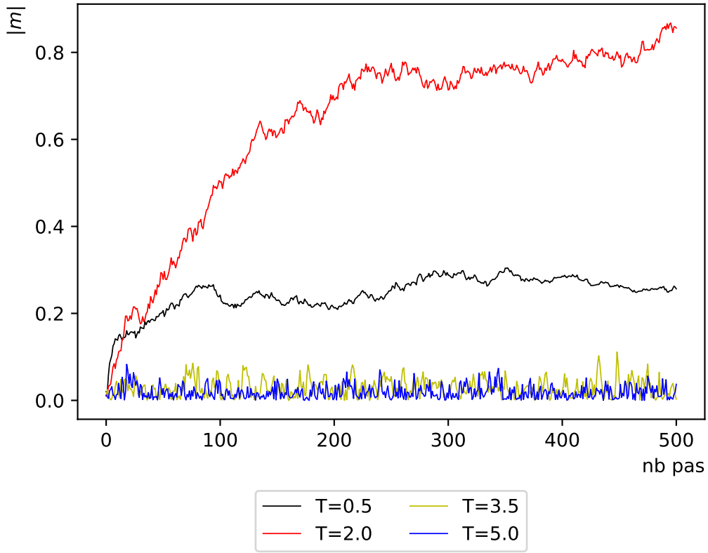
Evolution de l'Aimantation pour différentes températures sur 500 pas de Monte Carlo
